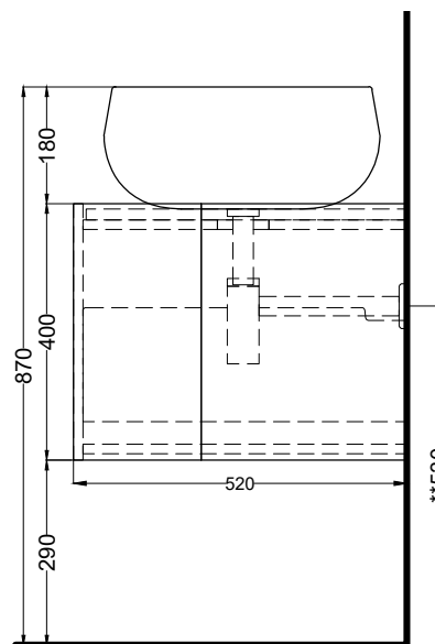
PROSPETTO LATERALE
