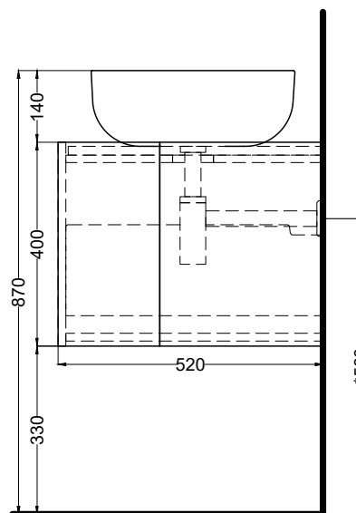
PROSPETTO LATERALE
