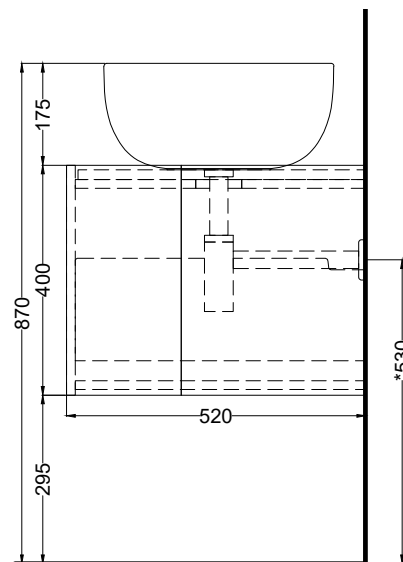
PROSPETTO LATERALE
