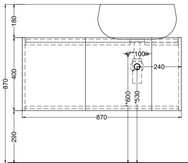
PROSPETTO FRONTALE
